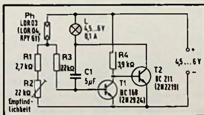
Bild 1. In dieser Multivibratorschaltung dient ein Fotowiderstand als Koppelglied. Bei ausreichendem Umlicht schaltet er den Blinkgeber ab
