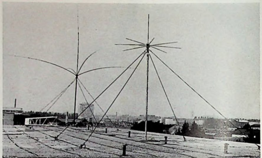
Bild 1. Aktive und – im Hintergrund – passive HF-Antennenanlage
