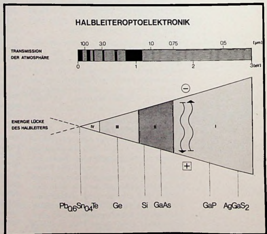
Bild 1. Zusammenhang zwischen Wellenlänge der Strahlung und der Energielücke verschiedener Halbleitermaterialien.
