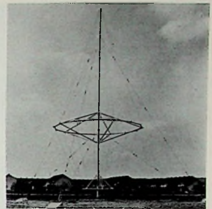
Bild 4: HF-Reusenantenne
