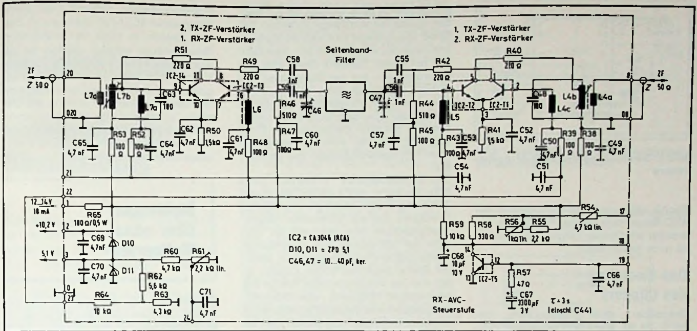
Bild 4. Platinschaltung des SSB-ZF-Aufbereiters
