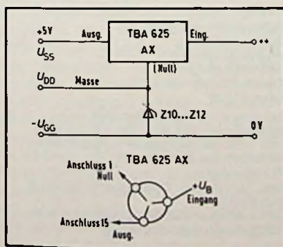
Bild 3. Spannungsstabilisierung für den Netz-Betrieb des Geräts
